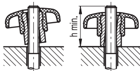
Anwendungsbeispiele Der Gewindebolzen muss länger als "h" sein
